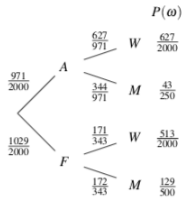
Inverses Baumdiagramm:
